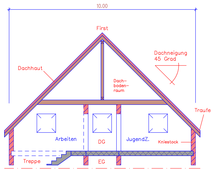
Einfacher Schnitt durch das DG und Dachspitz
